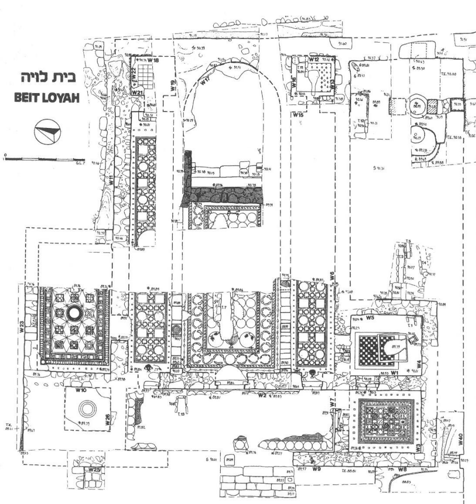
בית לוייה; תכנית כללית של הכנסייה ושל המיתקנים שלידה
