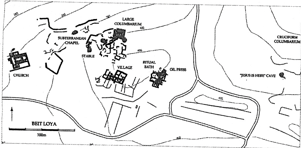
3 חורבת בית לוייה - תוכנית כללית
